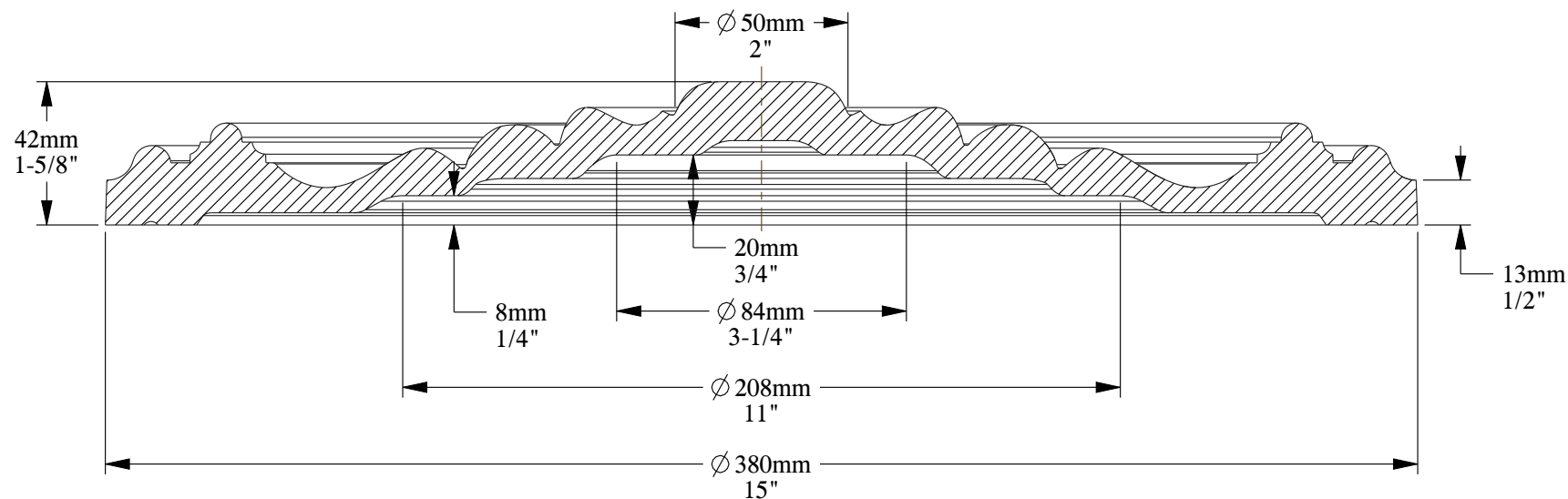
SECTION A-A SCALE 1:2
