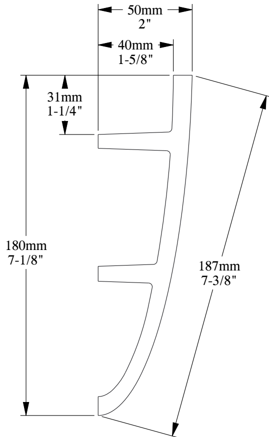
SCALE 1:2
