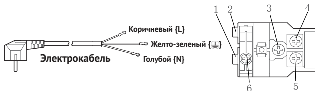
КЛЕММНАЯ КОРОБКА
