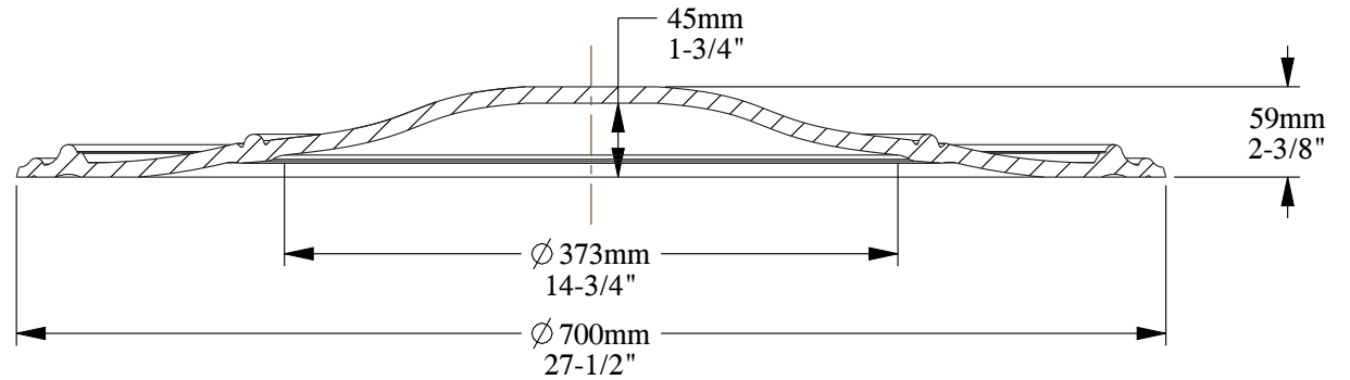
SECTION A-A SCALE 1:5
